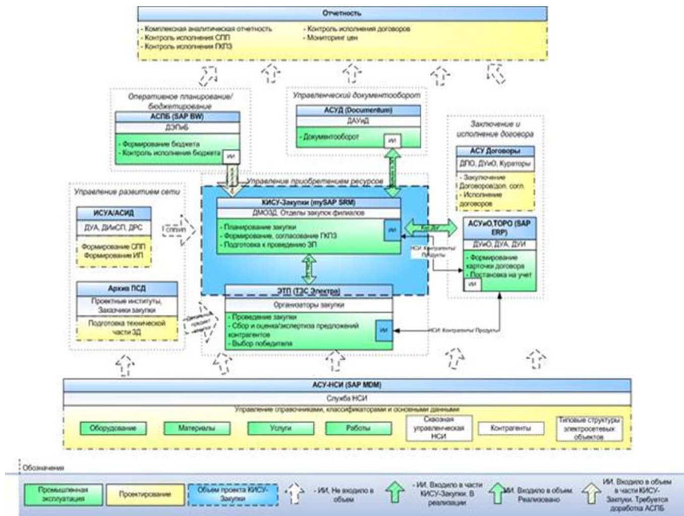
Рис.1 Архитектура решения АС «КИСУ-Закупки»
